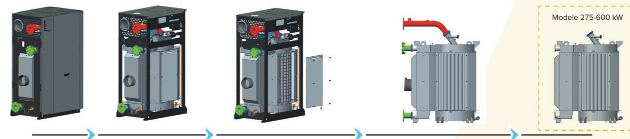
Demontaż obudowy
