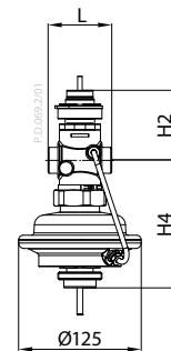
AVQMT PN 25 DN 15-50
