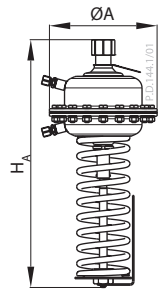
AFD 2 Actuator
