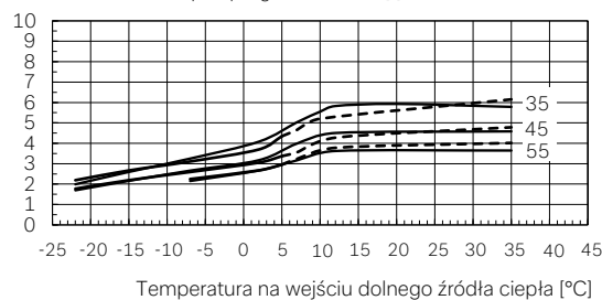
COP z udziałem pomp wg EN 14511 w [-]
