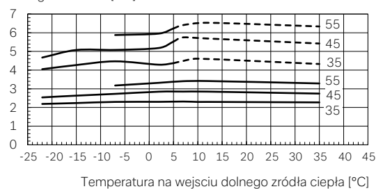
Pobór mocy elektrycznej z udziałem pompy i wentylatora wg EN 14511 [kW]
