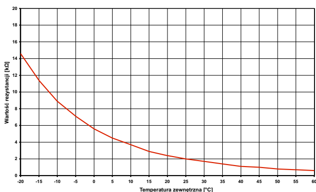
Abb. 3.4: Charakterystyka czujnika NTC-2 zgodnego z normą DIN 44574
