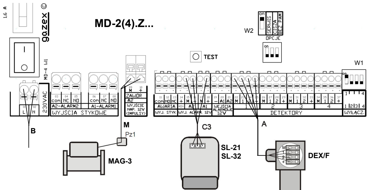
Rys.3.2 Widok poglądowy komory zaciskowej modułu i połączeń przewodowych
