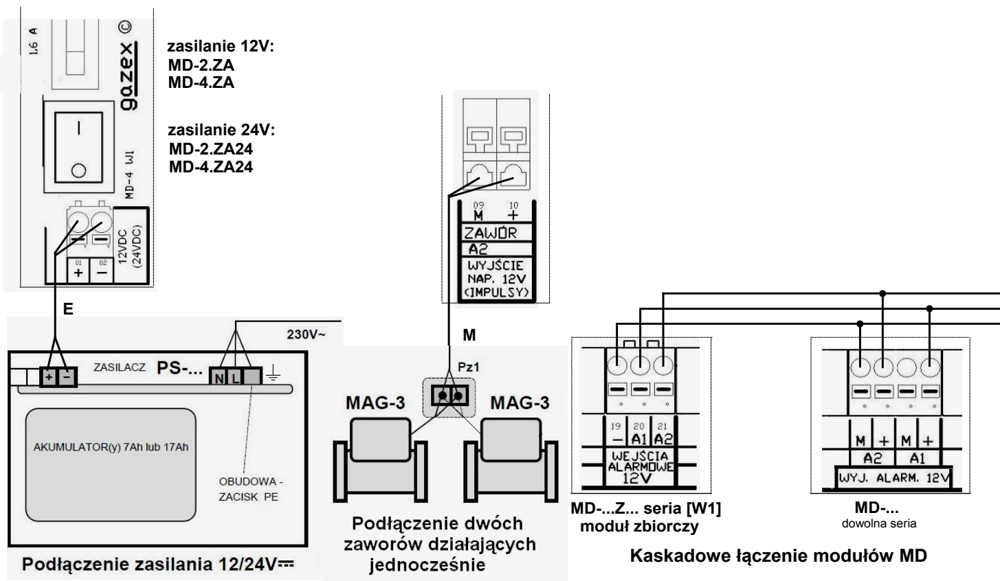
Rys.3.2.A Połączenia przewodowe różnych wariantów systemu
