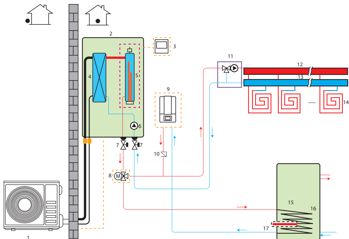
Rysunek 2.1.4.1: Ogrzewanie pomieszczeń i ciepła woda użytkowa z dodatkowym źródłem ciepła zapewniającym tylko ogrzewanie pomieszczeń
