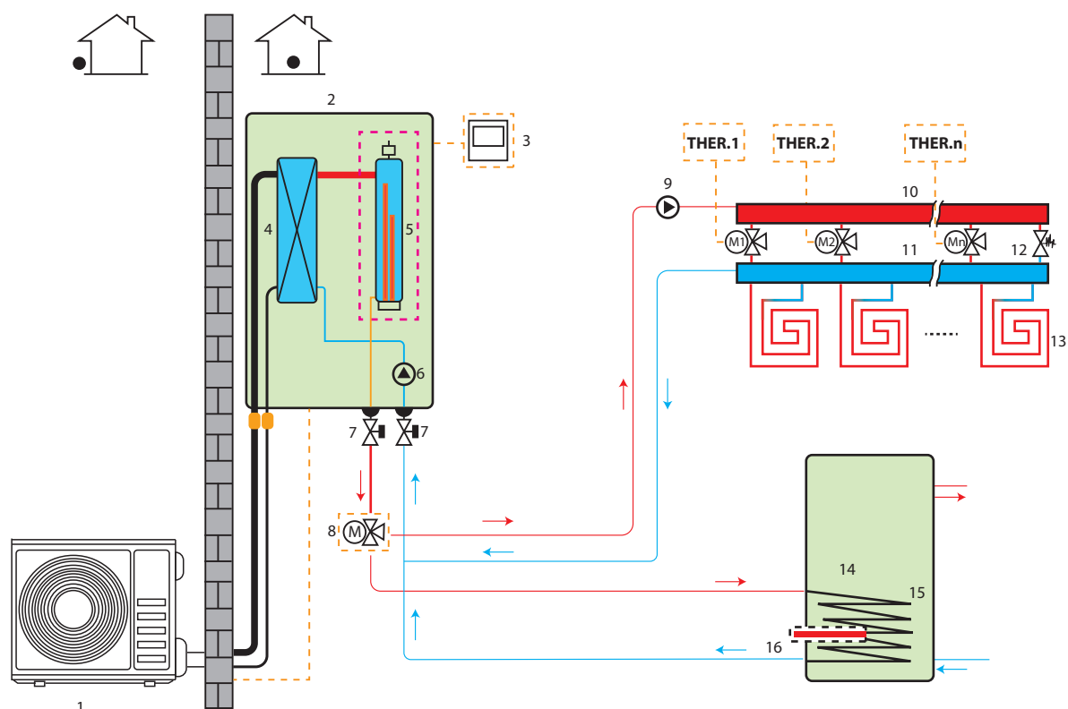
Rysunek 2.1.2: Ogrzewanie pomieszczeń i ciepła woda użytkowa
