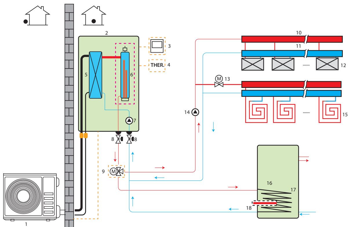
Rysunek 2.1.3: Ogrzewanie pomieszczeń, chłodzenie pomieszczeń i ciepła woda użytkowa
