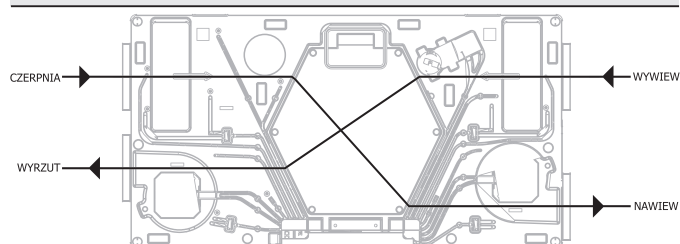
Schemat zasady działania wymiennika przeciwprądowego dla Alternatywnej (B) wersji wykonania.
