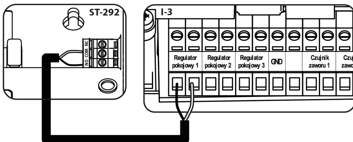
Przykładowe podłączenie regulatora dwustanowego
