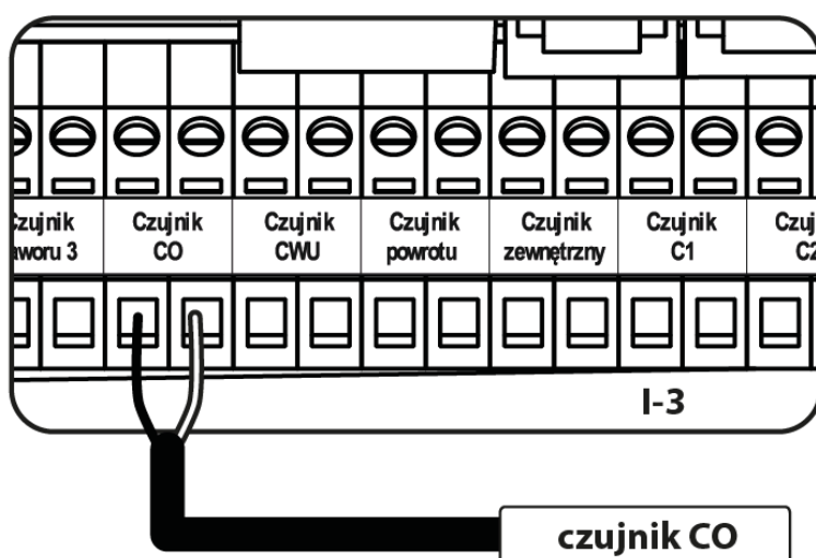
Podłączenie czujnika CO
