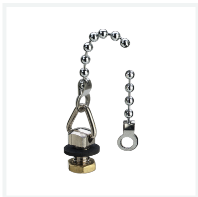
Łańcuszek kulkowy wyposażenie Wspornik z łańcuszkiem nr wzoru 9928.190
