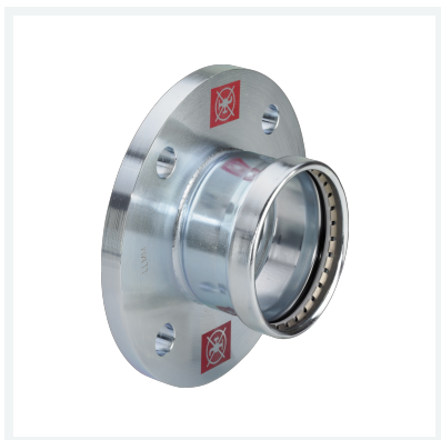
Prestabo XL-przejsie kołnierzowe z SC-Contur nr wzoru 1159.1XL nr kat. 629 915
