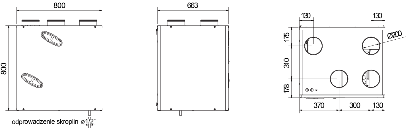
Schemat podłączenia przewodów wentylacyjnych do rekuperatora Reversus 600+
