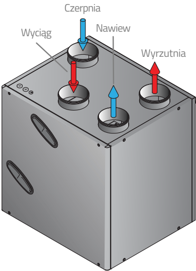
Schemat podłączenia przewodów wentylacyjnych do rekuperatora Reversus 600+
