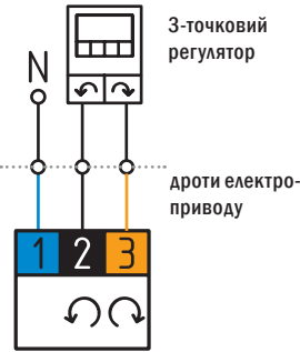
Рис. 6. Схема 3-точкового електричного привиду
