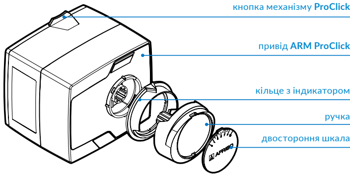
Рис. 1. Конструкція привиду ARM ProClick
