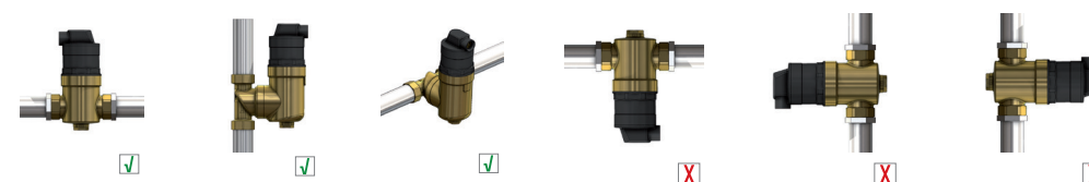
Rys. 4. Dopuszczalna pozycja montażowa separatora powietrza AAS
