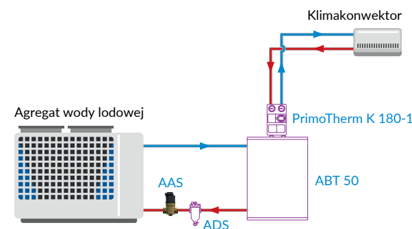
Rys. 3. Przykładowe schematy instalacji z separatorem powietrza AAS
