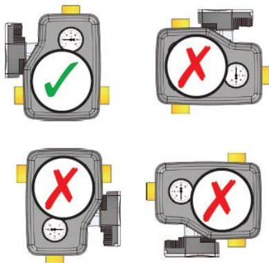
Rysunek 5: Dopuszczalne pozycje montażowe grup pompowych RTA
