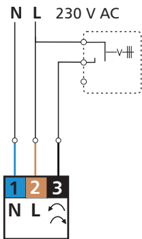
AZV electrical diagram / Schemat elektryczny AZV / Elektroschaltplan AZV / Schéma électrique AZV / Электрическая схема AZV
